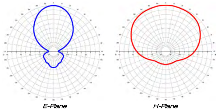
E-Plane
