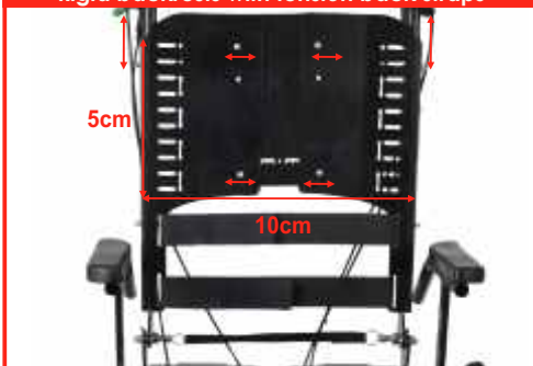
Respaldo rígido con fajas tensoras Rigid backrests with tension back straps
