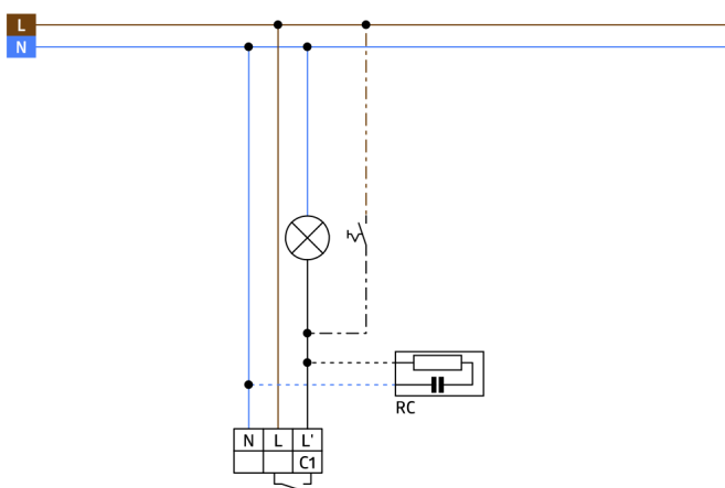
Wiring diagrams
