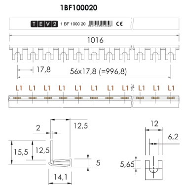
Dim. em mm
