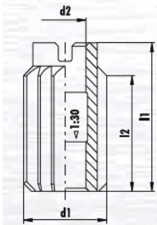
Aufsteckreibahlen HSS-E, DIN 219 Shell Reamers HSS-E, DIN 219
